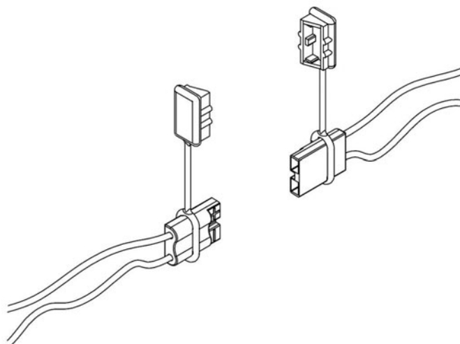
Ensemble de fils connecteur pour démarrage électrique:
