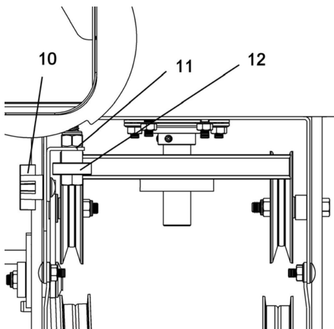
Positionner la fixation du roulement à billes
